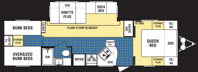
FS310B-DSL
